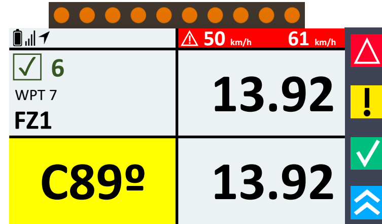
Foto 14. Display Zona de Velocidad Limitada – Velocidad Excesiva
