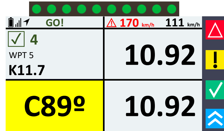
Foto 12. Display Solicitud Adelantamiento – Adelantamiento Confirmado
