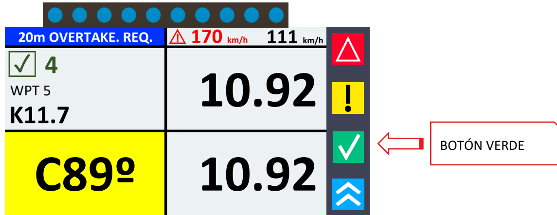
Foto 11. Display Solicitud Adelantamiento – Adelantamiento Solicitado
