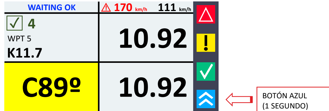
Foto 10. Display Solicitud Adelantamiento – Esperando Confirmación
